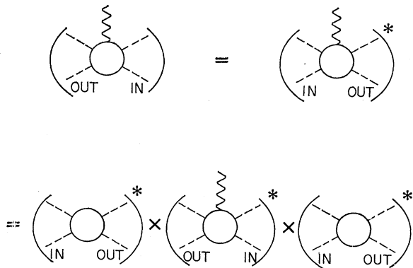
FIG. 8. Phase theorem for \pi\pi \rightarrow \pi\pi\gamma .
